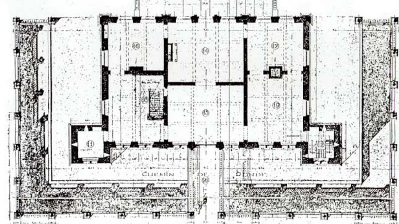
REZ-DE-CHAUSSEE.
