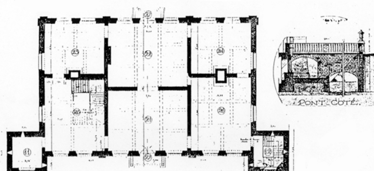
PREMIER ETAGE.
